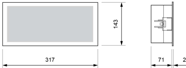
Flush mounting (corte: 300 x 127 mm)
